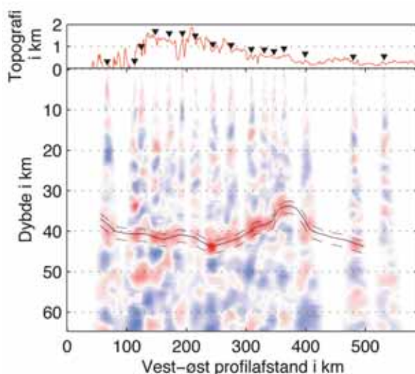
Figur 4: Øverste del: topografi (rød linje) og seismografpositioner (sorte trekanted) langs profillinjen på figur 2. Nederste del: et lodret tværsnit af jordskorpen langs profillinjen. Områder med kraftig rød farve angiver laggrænser. Skorpens underside er tolket med en tynd sort linje. Usikkerheden på tolkningen fra estimeret hastighedsmodel er angivet med de stiplede linjer.
