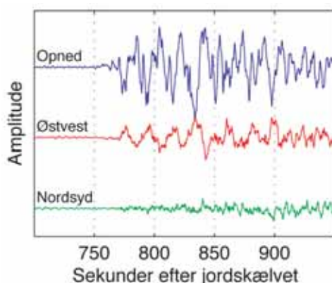
Figur 1: Registrering af jordens forskydning i 3 retninger for P-bølgen fra 9,0-skælvet ved Sumatra registreret på en seismograf i Mønsted kalkmine. Signalet på nord-syd-komponenten er meget svagt, da skælvet ligger i øst.
