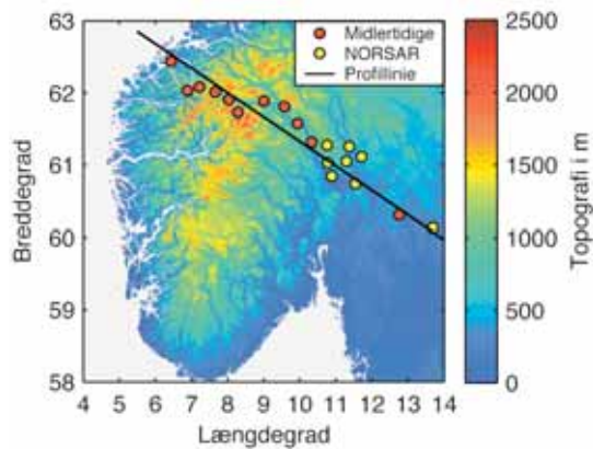
Figur 2: Sydnorges topografi samt positionen af de midlertidige og permanente (NORSAR) seismografer. Linjen angiver tværsnittet vist på figur 4.
